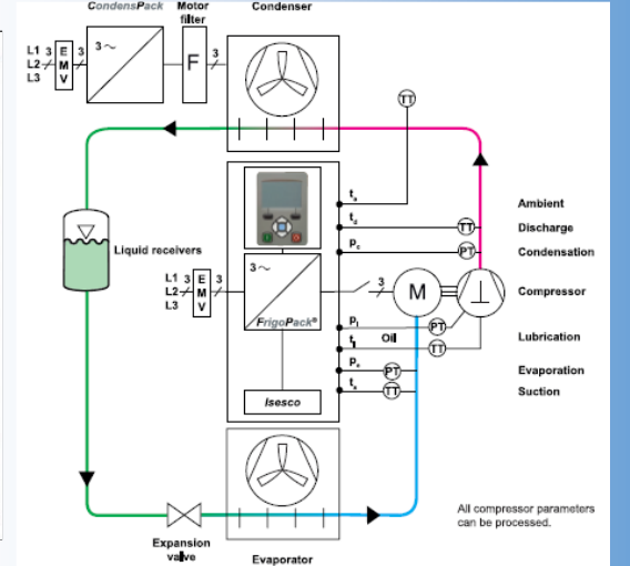
FrigoPack kontrol ile soğutma çevrimi
